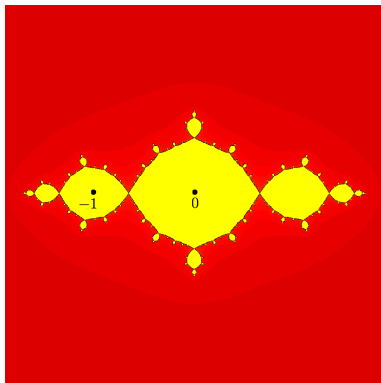
Figura 8: El pla de fases de F(z) = z^2 - 1 . L’òrbita \{0, -1\} és 2-periòdica i atractor. En groc es veu la seva conca d’atracció, part del conjunt de Fatou. En vermell es veu la conca d’atracció del punt de l’infinít. La frontera comuna de les dues conques és el conjunt de Julia.
