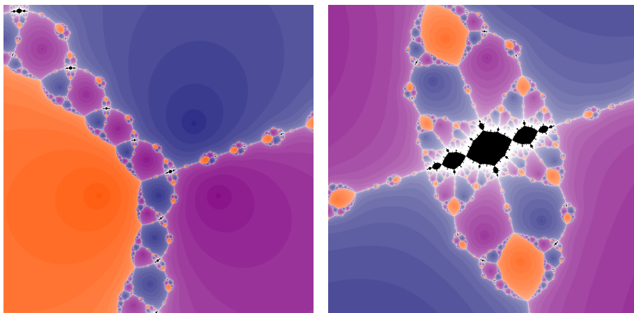
Figura 14: Esquerra: El pla de fases del mètode de Newton del polinomi P(z) = z(z-1)(z-a) amb a escollit adequadament. Dreta: Una ampliació on veiem un dels conjunts de condicions inicials dolentes. En aquest cas concret, es tracta de la conca d'atracció d'una òrbita periòdica de període 2.
