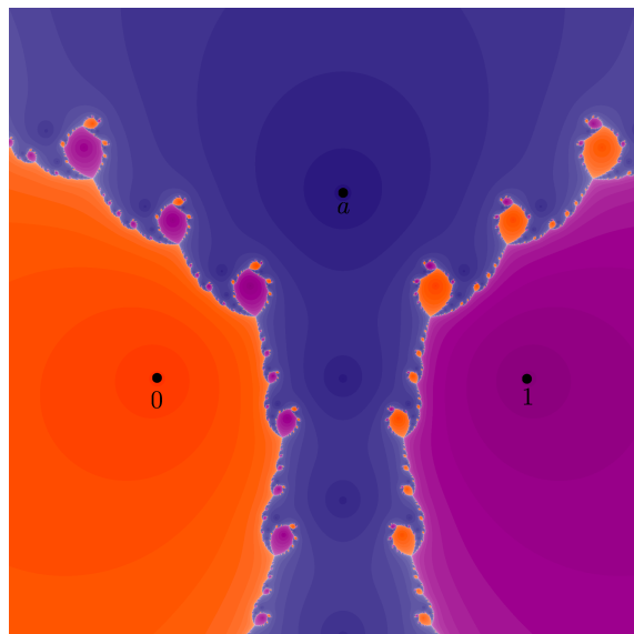
Figura 6: Pla dinàmic del mètode de Newton N_P per a P(z) = z(z-1)(z-a) amb a = \frac{1}{2}(1+i) . Veiem tres conques d'atracció totalment invariants. Una d'elles, la de a , està formada per un únic component connex mentre que les altres dues en tenen infinits.
