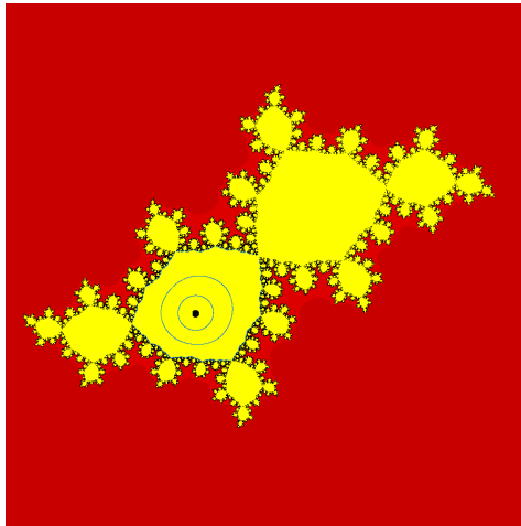
Figura 10: Pla de fases de F(z) = \lambda z(1 - z) on \lambda = e^{2\pi i \frac{1-\sqrt{5}}{2}} . En groc es mostra un disc fix de Siegel al voltant de z = 0 i totes les seves antiimatges. En vermell la conca d'atracció de l'infinit.
