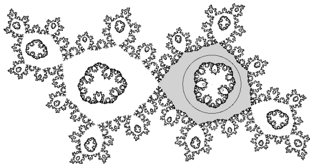
Figura 11: Pla de fases de F(z) = z^2 \frac{z-a}{1-\bar{a}z} per un cert valor de a escollit convenientment. En gris es mostra un anell de Herman, dins del qual hi ha dibuixada una de les seves corbes invariants
