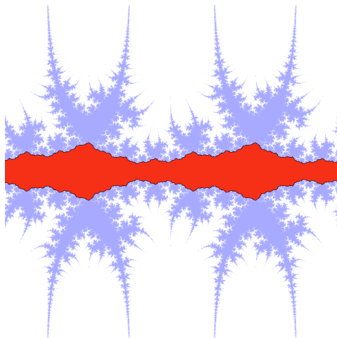
Figura 12: Pla de fases de F(z) = z + a + b \sin(z) amb a i b escollits adequadament per a que el conjunt de Fatou tingui un domini de Baker que es mostra en vermell. Les òrbites dins d'aquest domini tendeixen cap a l'infinit amb velocitat lineal. En blau veiem totes les antiimatges del domini de Baker.
